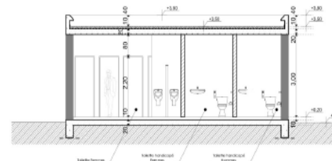
COUPE B-B
