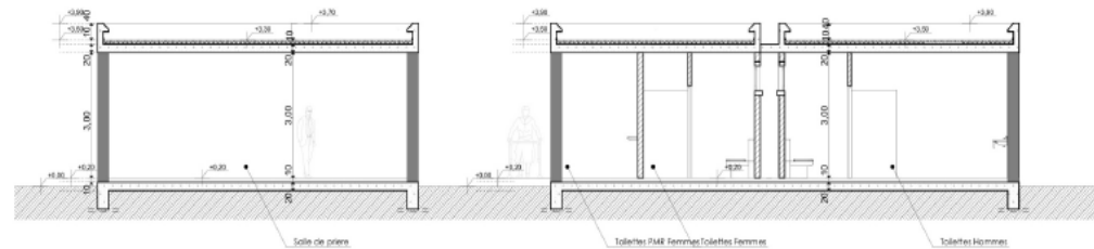
COUPE A-A
